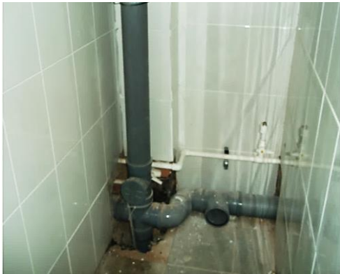
Отсутствует гидроизоляция в перекрытии - сложности в эксплуатации системы.
